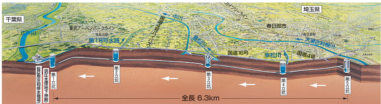
図-1 首都圏外郭放水路のイメージ図
