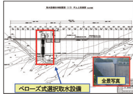
取水設備全体配置図
