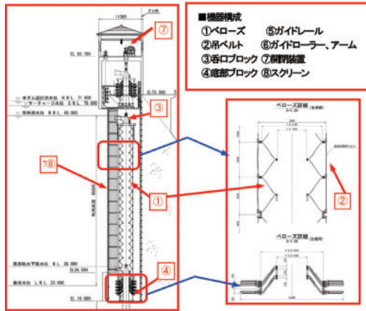
ベローズ式選択取水設備概要
