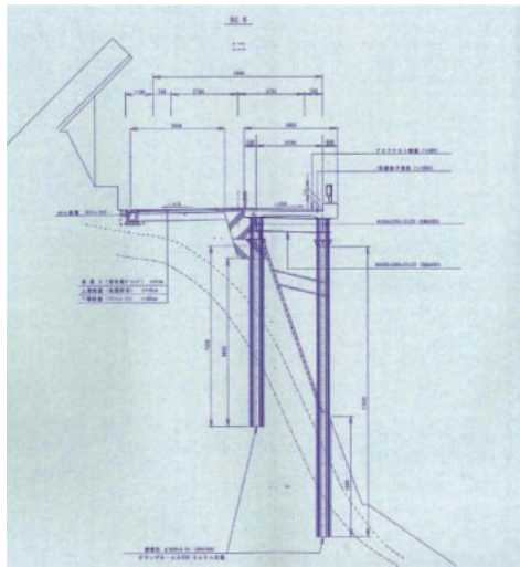
標準断面図
