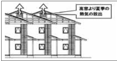
1号棟 東面立面図
