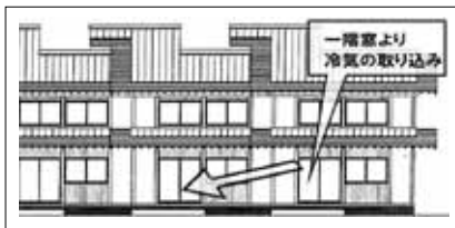
1号棟 南面立面図
