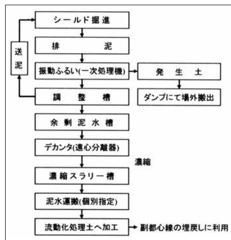
泥水再利用フロー図
