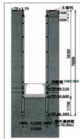
発進立坑断面図
